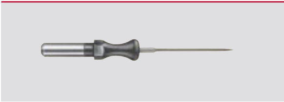
122-401-000 22 mm Nadelelektrode, gerade Needle electrode, straight Electrode à aiguille, droite Electrodo de aguja, recto Elettrodo a ago, retto
