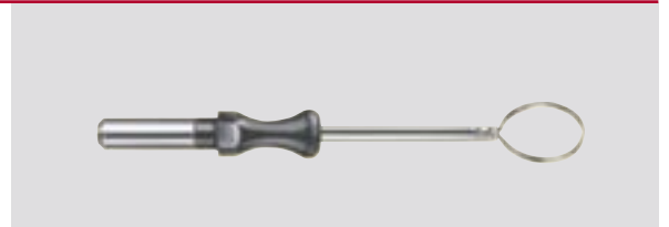
122-411-010 Ø 10 mm 0,2x0,6 mm Bandschlingenelektrode Ribbon loop electrode Electrode à bande métallique Electrodo de lazo de cinta Elettrodo a ansa a nastro
