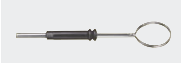
123-411-015 Ø 15 mm 0,2x0,6 mm Bandschlingenelektrode Ribbon loop electrode Electrode à bande métallique Electrodo de lazo de cinta Elettrodo a ansa a nastro
