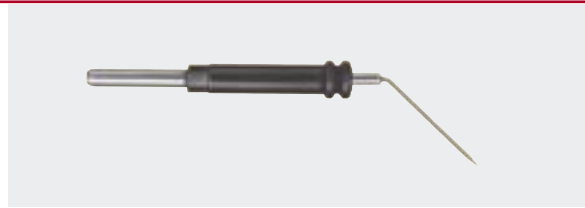
123-409-000 Nadelelektrode, 45° abgewinkelt Needle electrode, 45° angled Electrode à aiguille, coudée 45° Electrodo de aguja, acodado 45° Elettrodo a ago, curvo 45°
